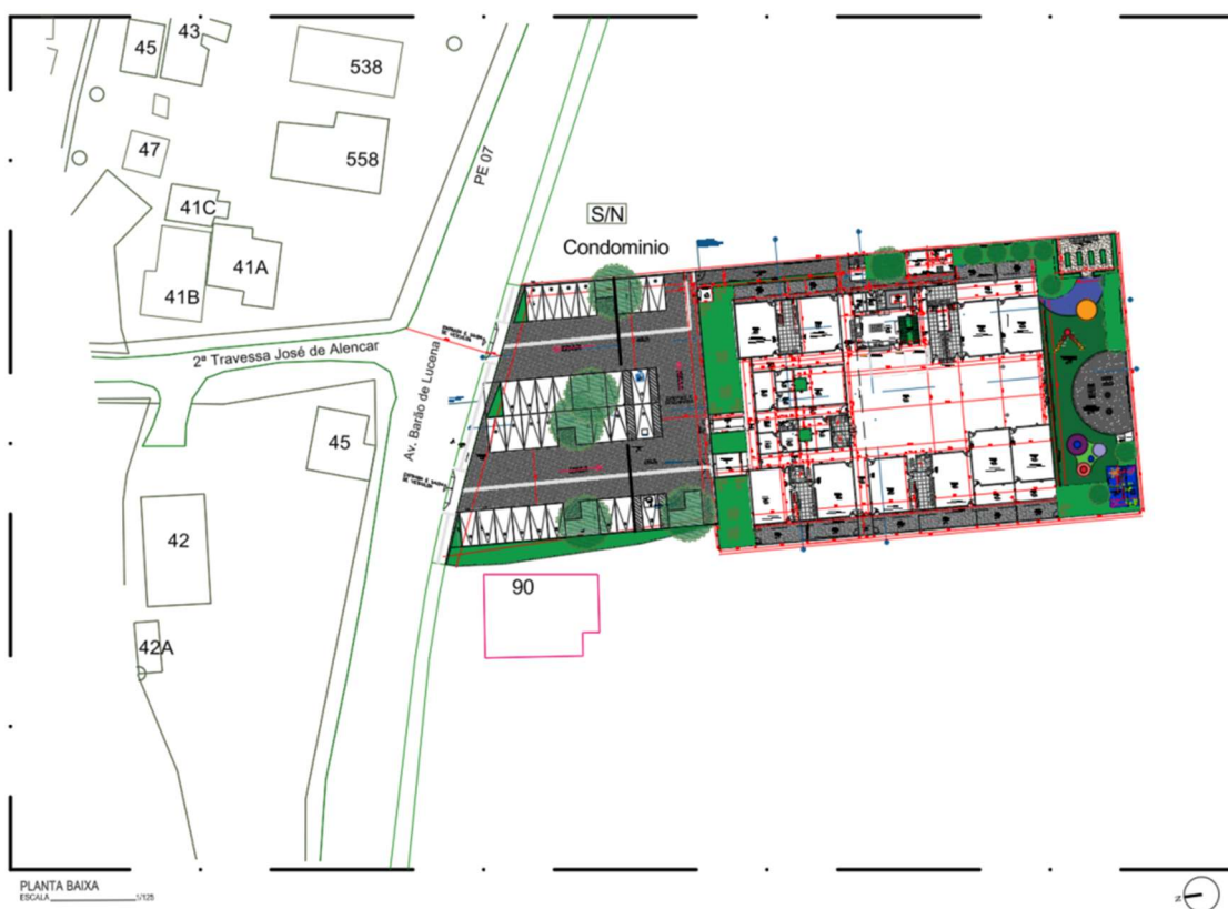
Figura 1: Planta baixa de implantação agenciamento da Creche 04, unidade Jaboatão dos Guararapes.
