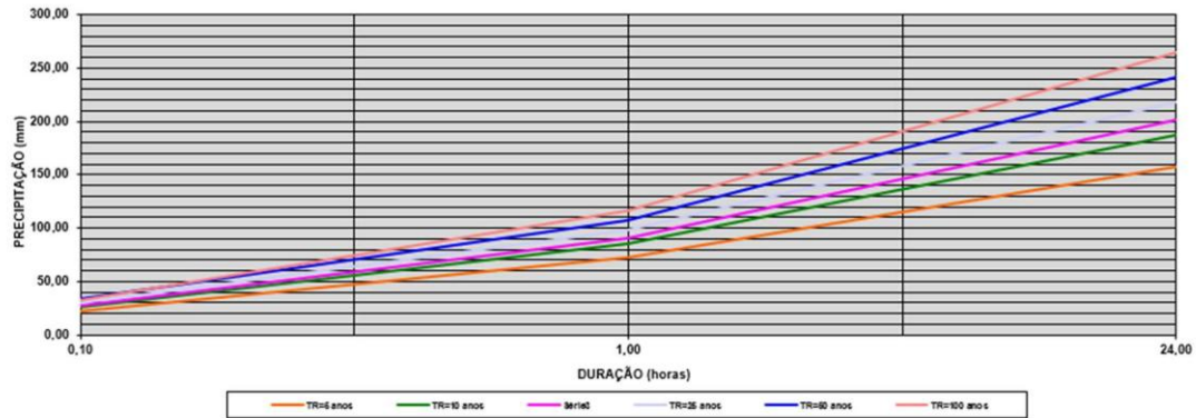
CURVAS DE PRECIPITAÇÃO X DURAÇÃO X FREQUÊNCIA
