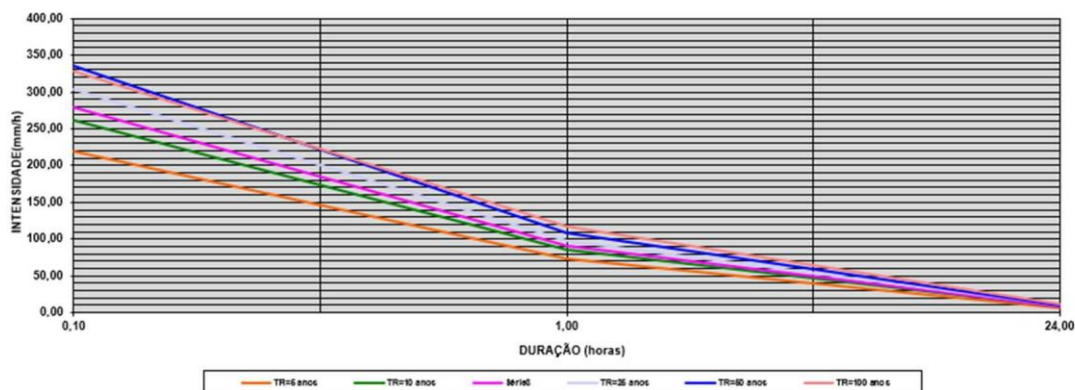
CURVAS DE INTENSIDADE X DURAÇÃO X FREQUÊNCIA
